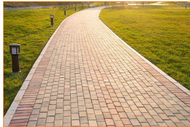
Устройство пешеходной дорожки из брусчатки
